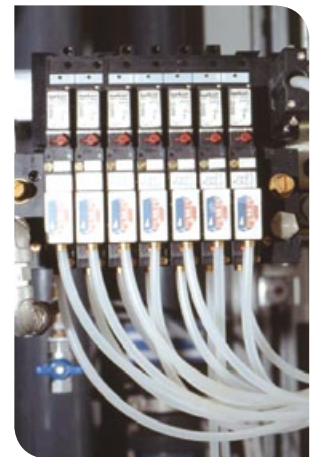
Druckluftsteuerung im Wasserwerk Karsdorf.
